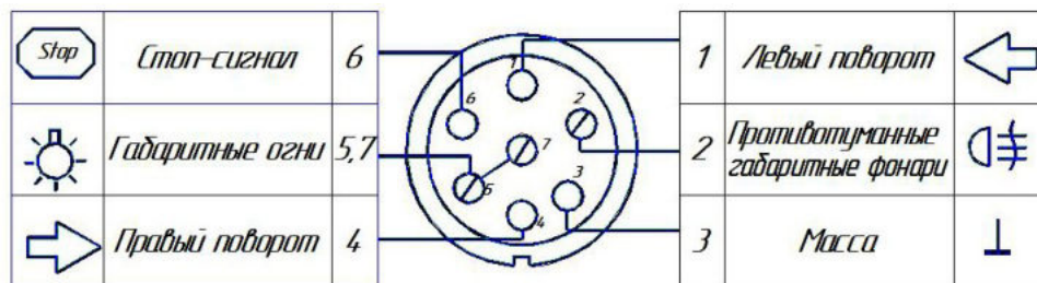
Схема подключения электрооборудования
