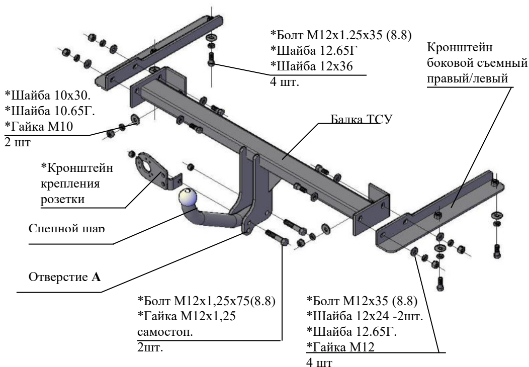
Рис.1 Тягово-сцепное устройство 9931
