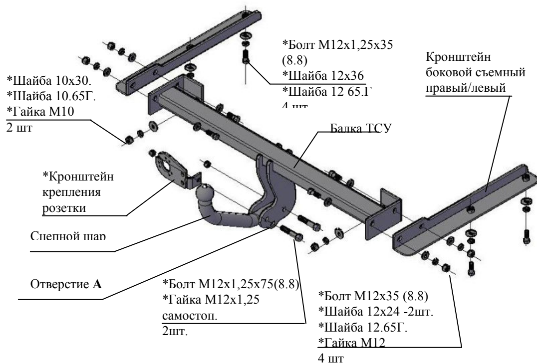
Рис.1 Тягово-сцепное устройство 9930
