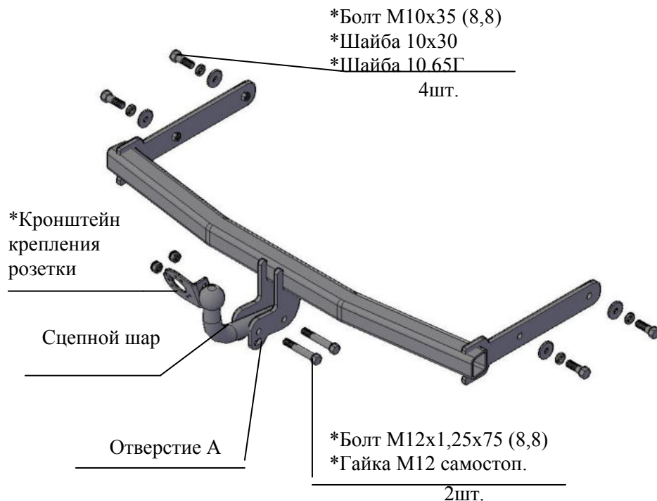
Рис.1 Тягово-сцепное устройство ТСУ 9731
