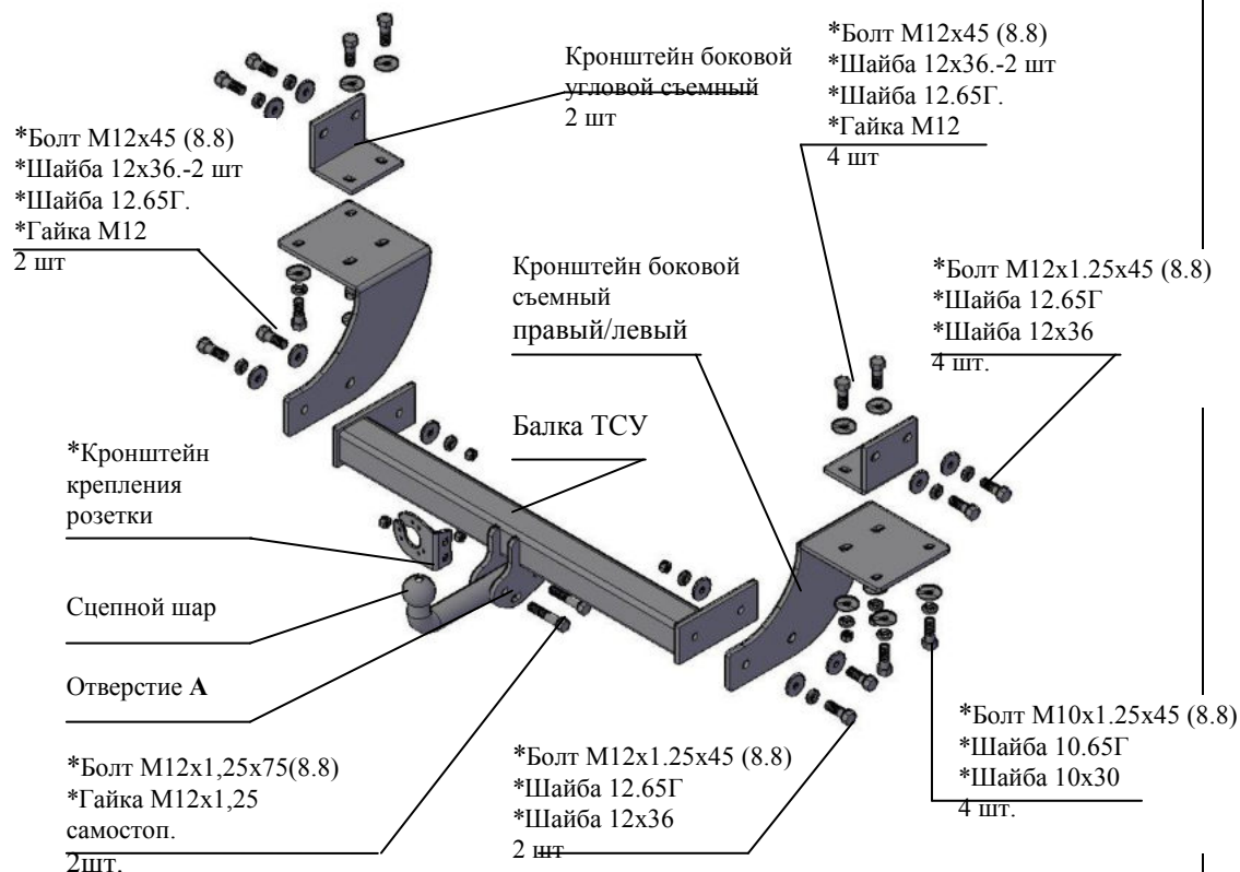
Рис.1 Тягово-сцепное устройство 9460
