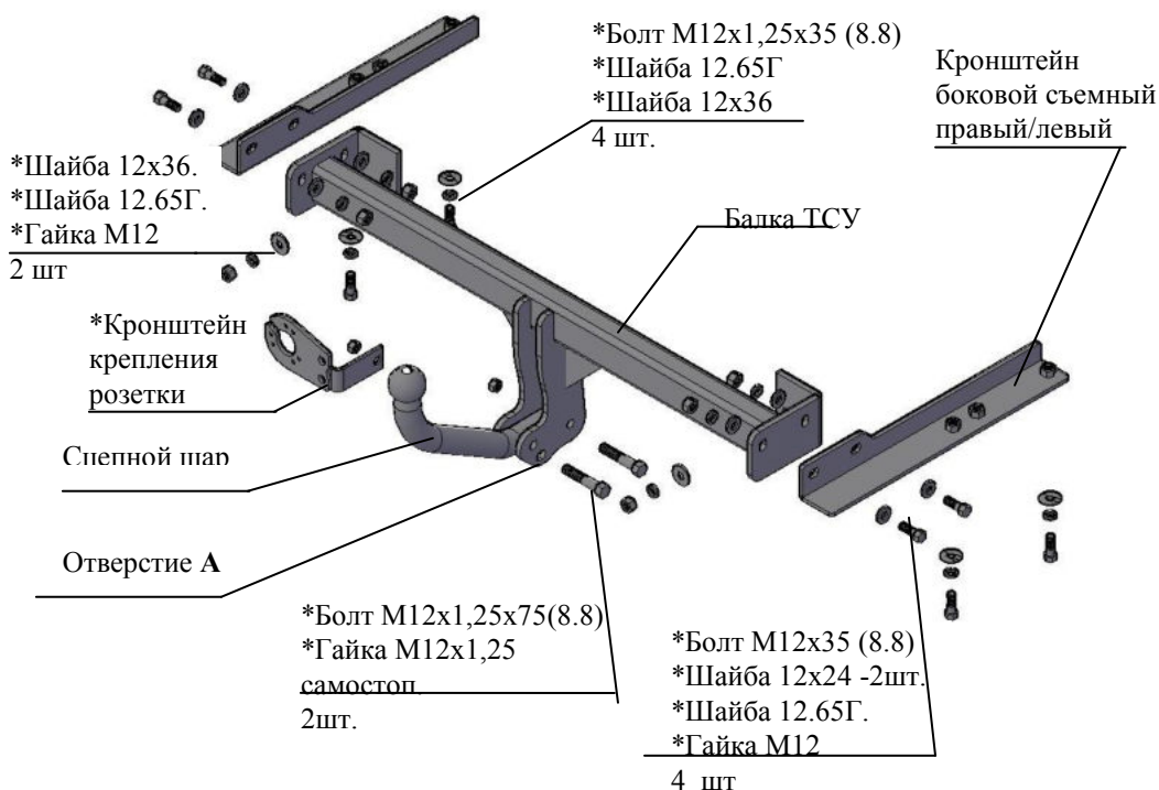
Рис.1 Тягово-сцепное устройство 9450
