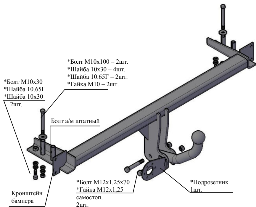
Рис.1 Тягово-сцепное устройство 9421
