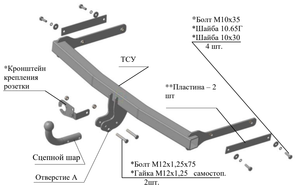
Рис.1 Тягово-сцепное устройство ТСУ 9151.
