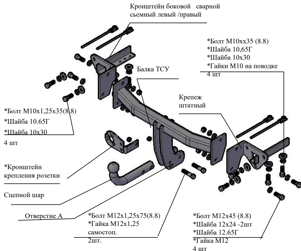
Рис.1 Тягово-сцепное устройство 8501 .
