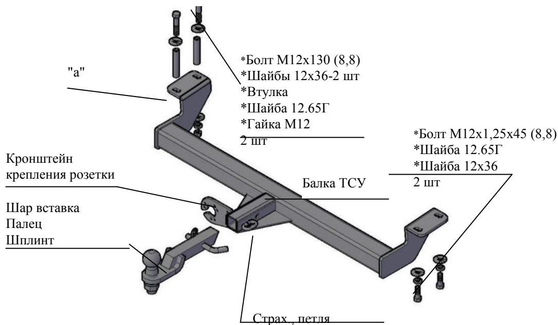
Рис.1 Тягово-сцепное устройство 8221.
