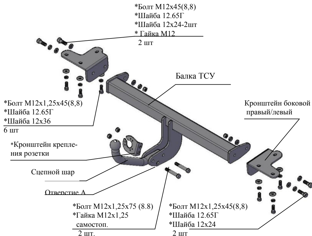
Рис.1 Тягово-сцепное устройство 7900.
