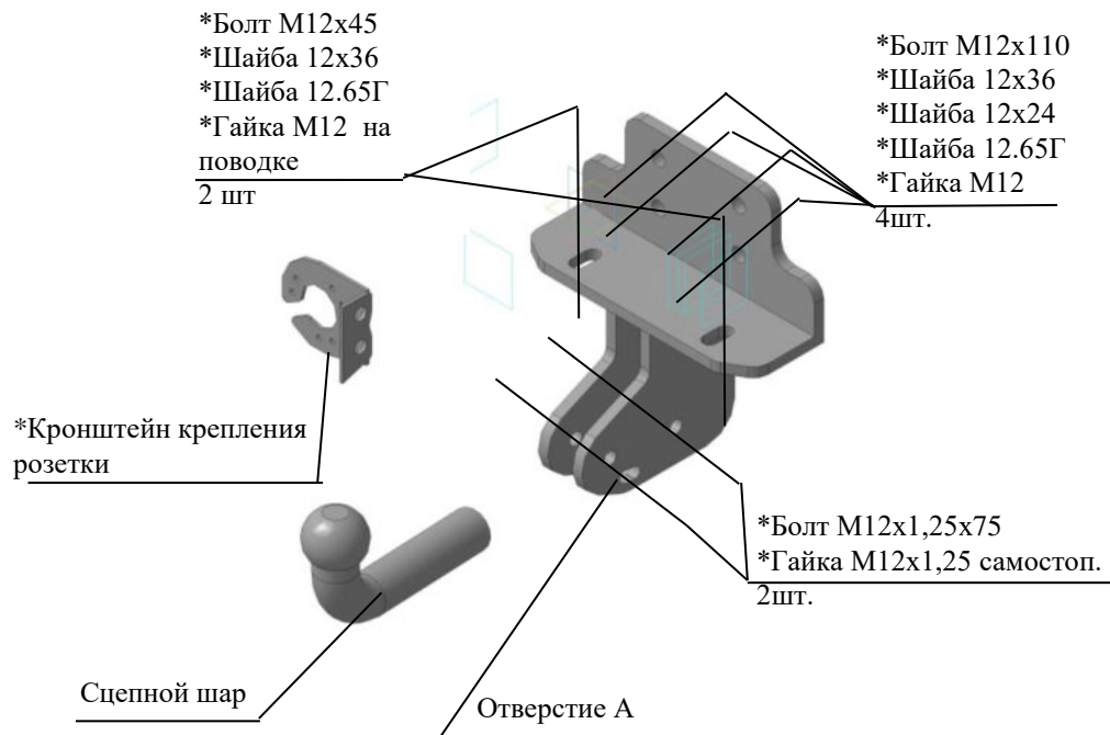
Рис.1 Тягово-сцепное устройство 7821.
