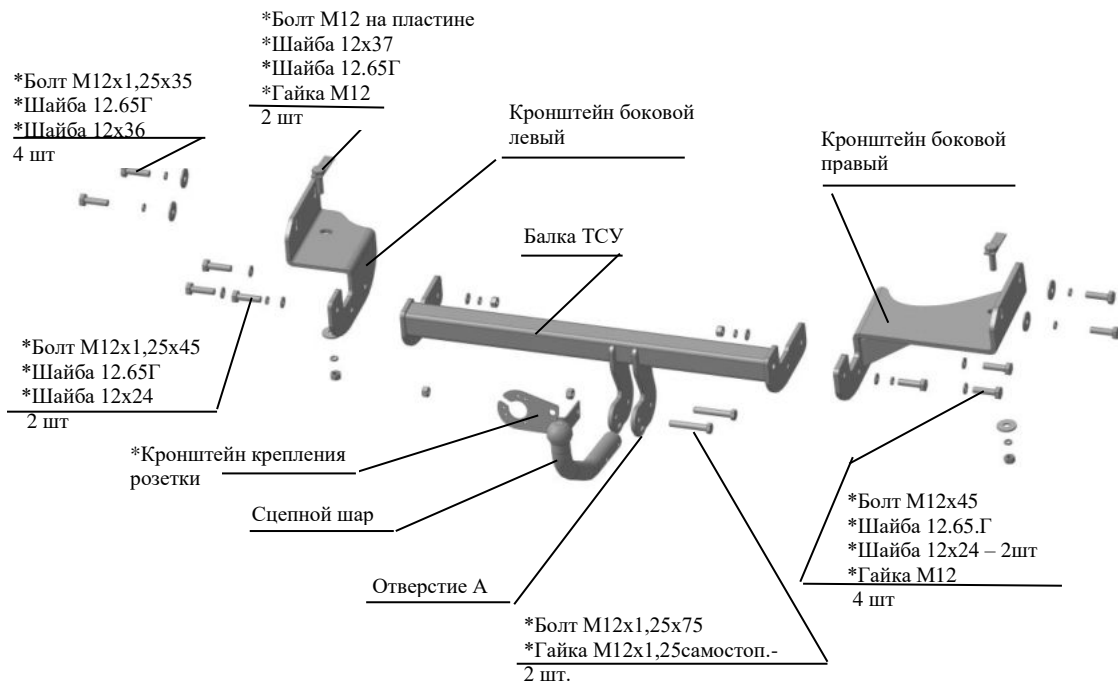
Рис.1 Тягово-сцепное устройство 7332
