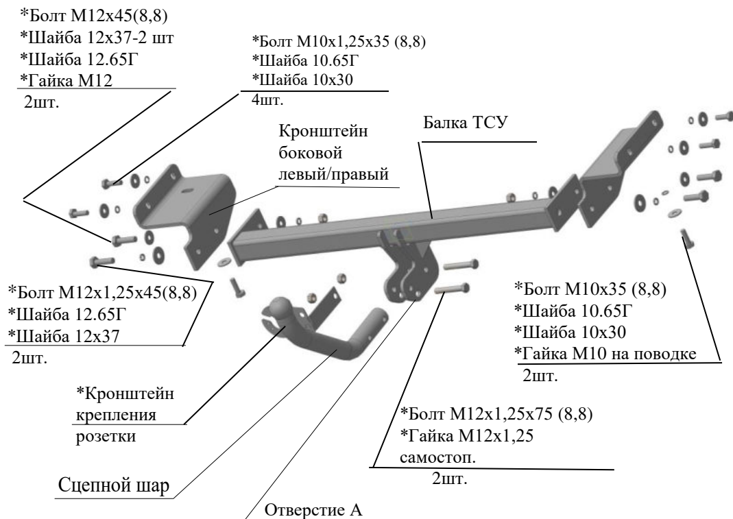
Рис.1 Тягово-сцепное устройство ТСУ 7260.
