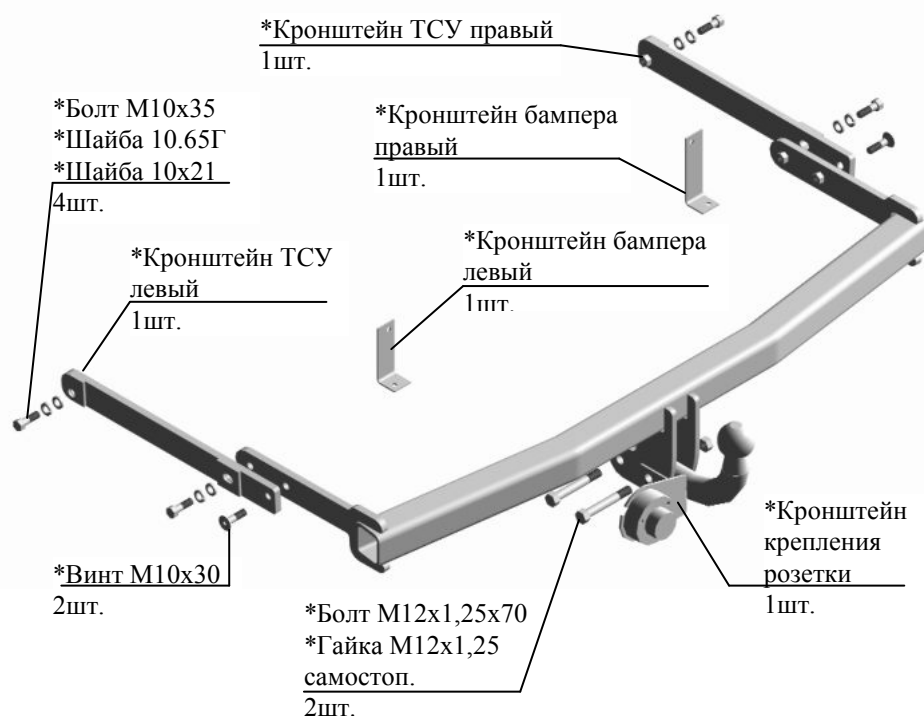
Рис.1 Тягово-сцепное устройство 6030
