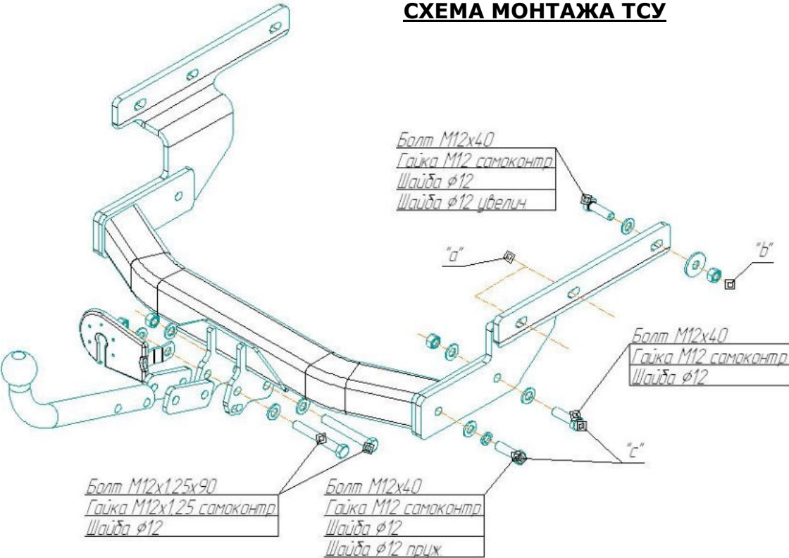
СХЕМА МОНТАЖА ТСУ
